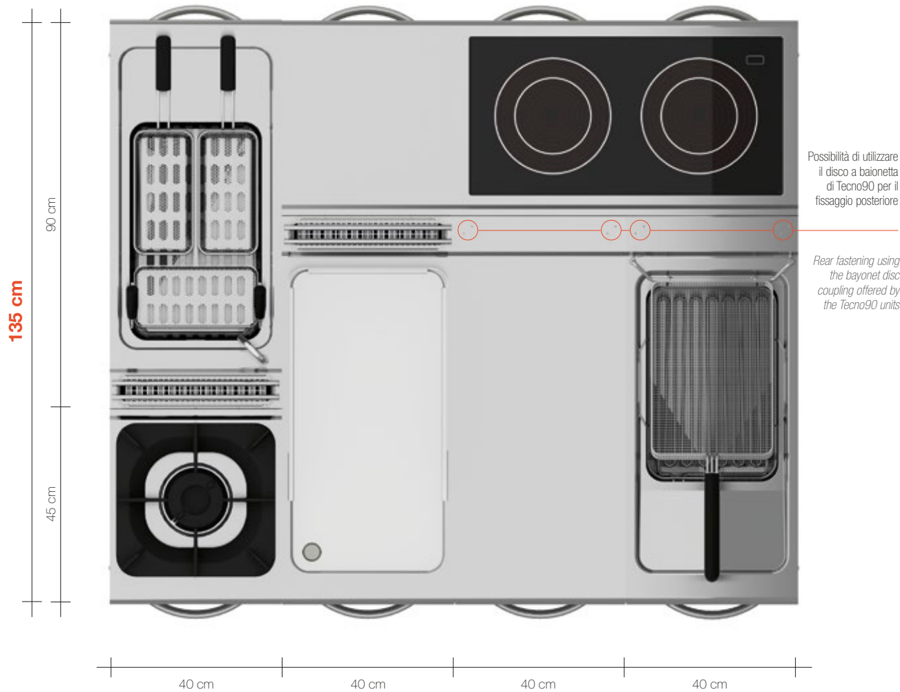
ISOLA CENTRALE MOSAICO IN COMPOSIZIONE CON TECNO90 MOSAICO CENTRAL ISLAND FEATURING THE TECNO90 LINE
